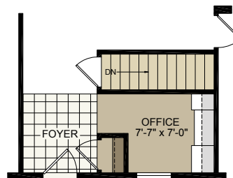
OPTIONAL STAIRWELL
