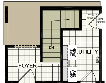
OPTIONAL BASEMENT
